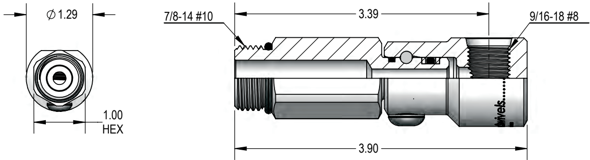
9 SS 4 MO 10 X FO 6 - 001 - Z - V
